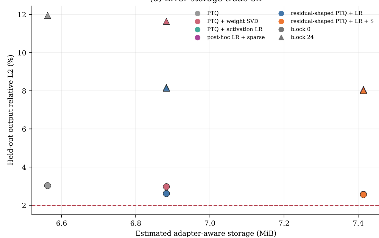
(d) Error-storage trade-off
