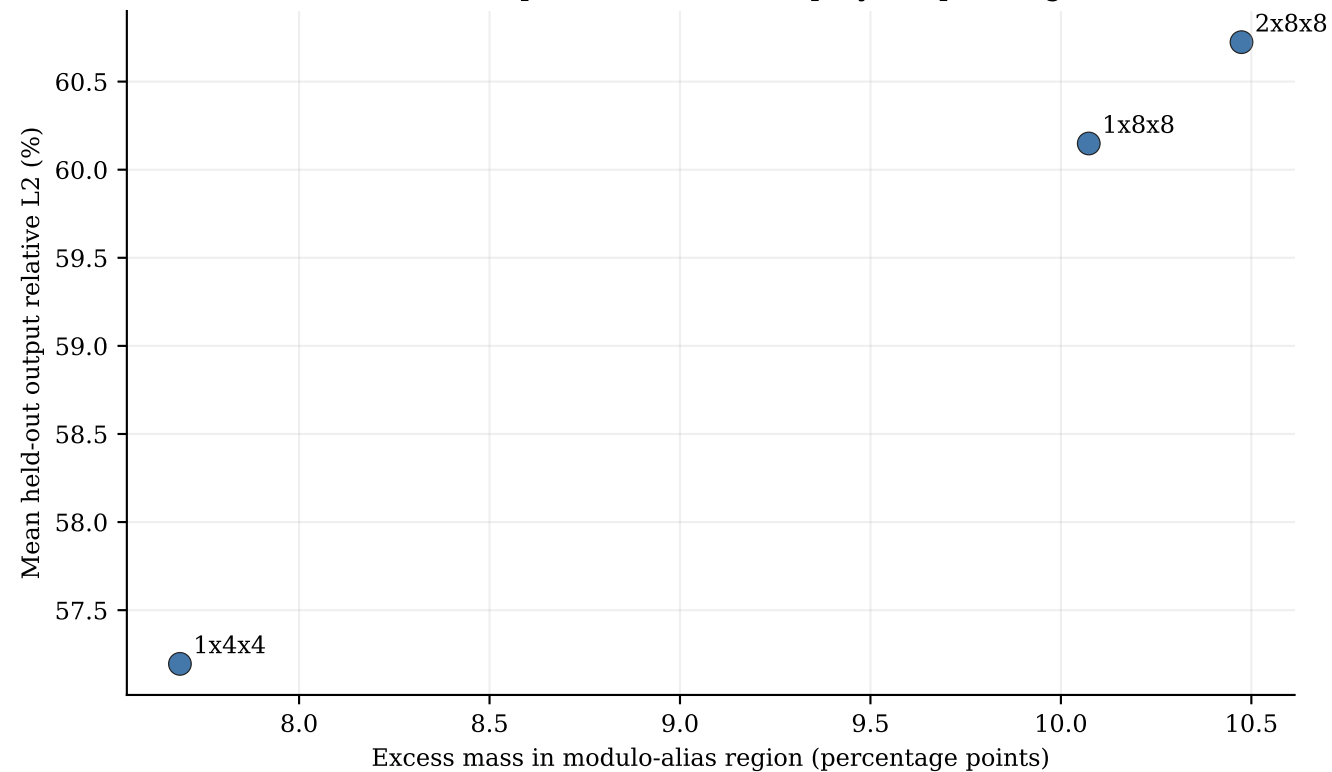
(d) Coarser periodic kernels amplify wrap leakage
