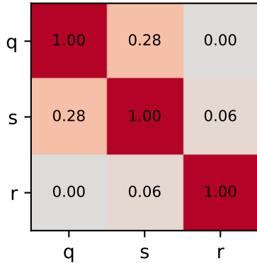
fc1
