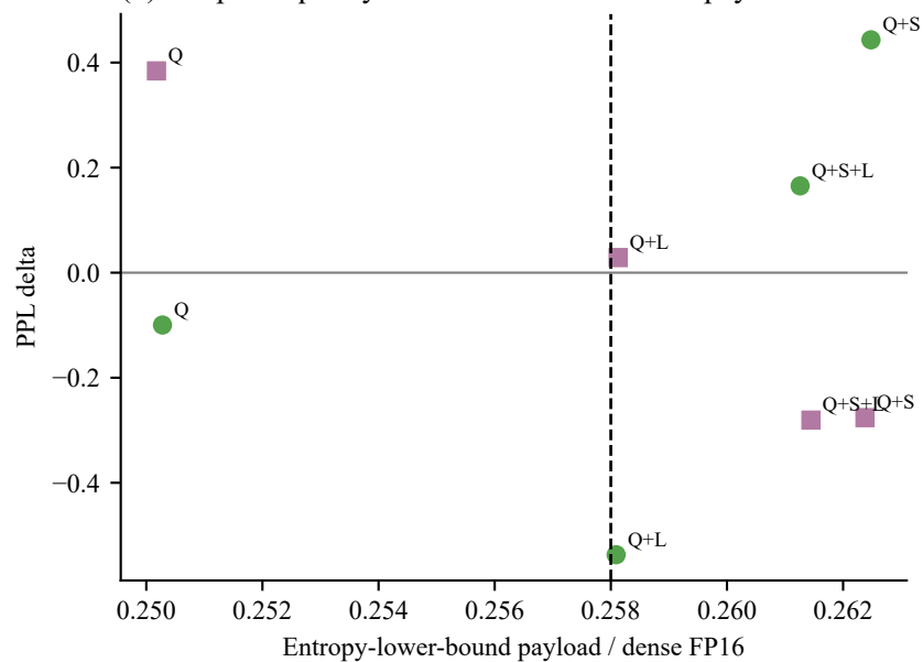
(d) Endpoint quality must be read with actual payload
