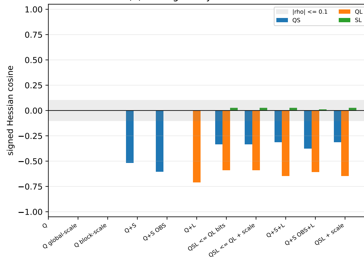
(d) Orthogonality vs cancellation
