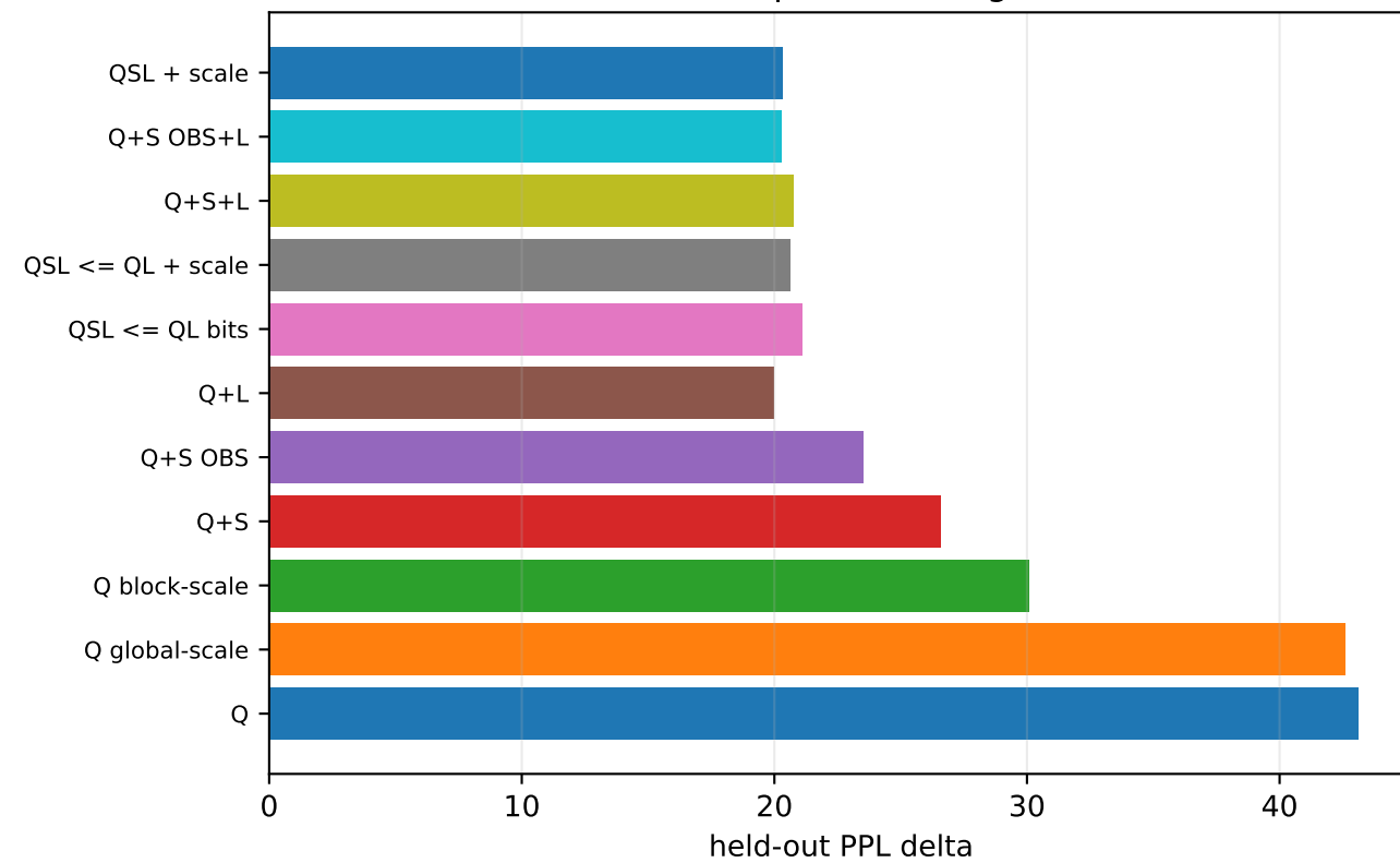
(d) Orthogonality vs cancellation
