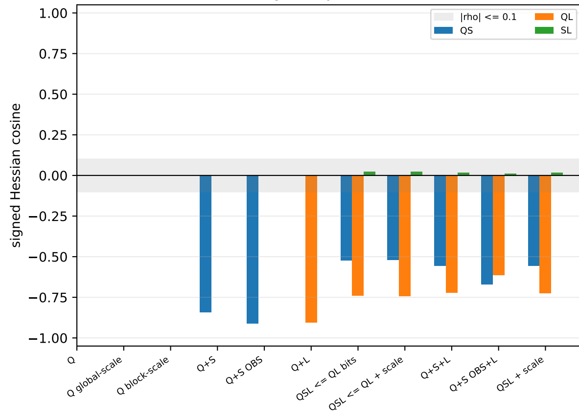
(d) Orthogonality vs cancellation
