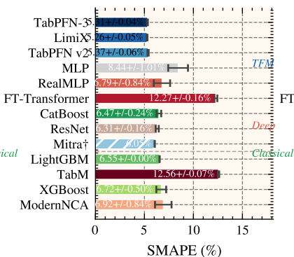
Matbench YS*
