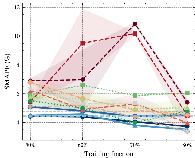
Matbench YS*
