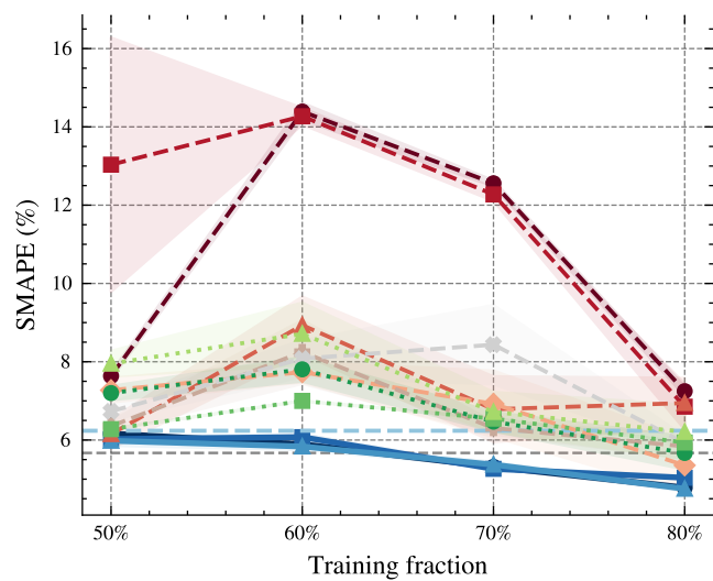
Matbench YS*
