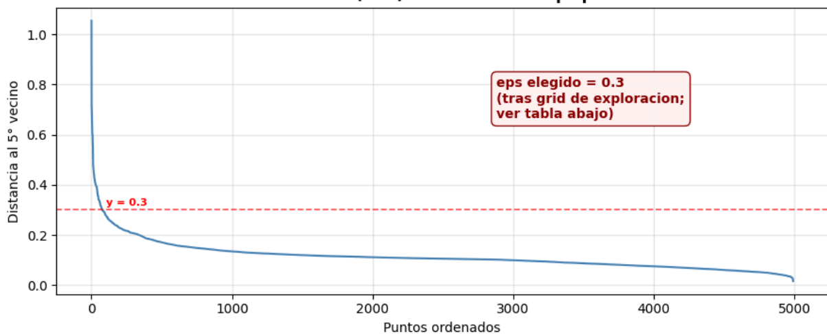
Gráfico k-distancia (k=5) — selección de eps para DBSCAN
