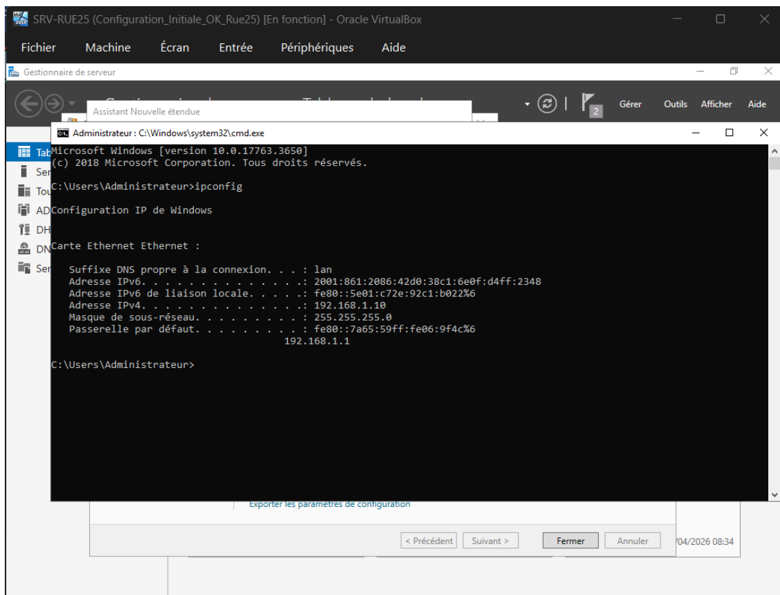
Figure 2 : Test de validation de l'adresse IP du serveur via la commande ipconfig.
