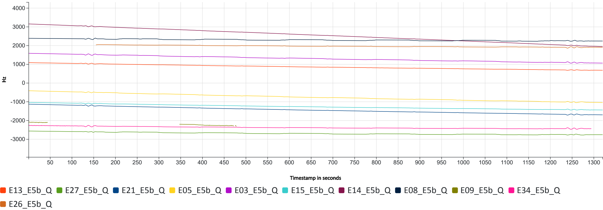
Doppler (hz) - Galileo E5b
