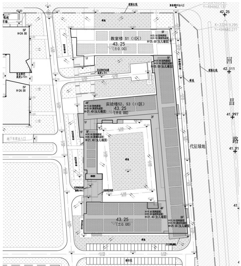
总平面图
