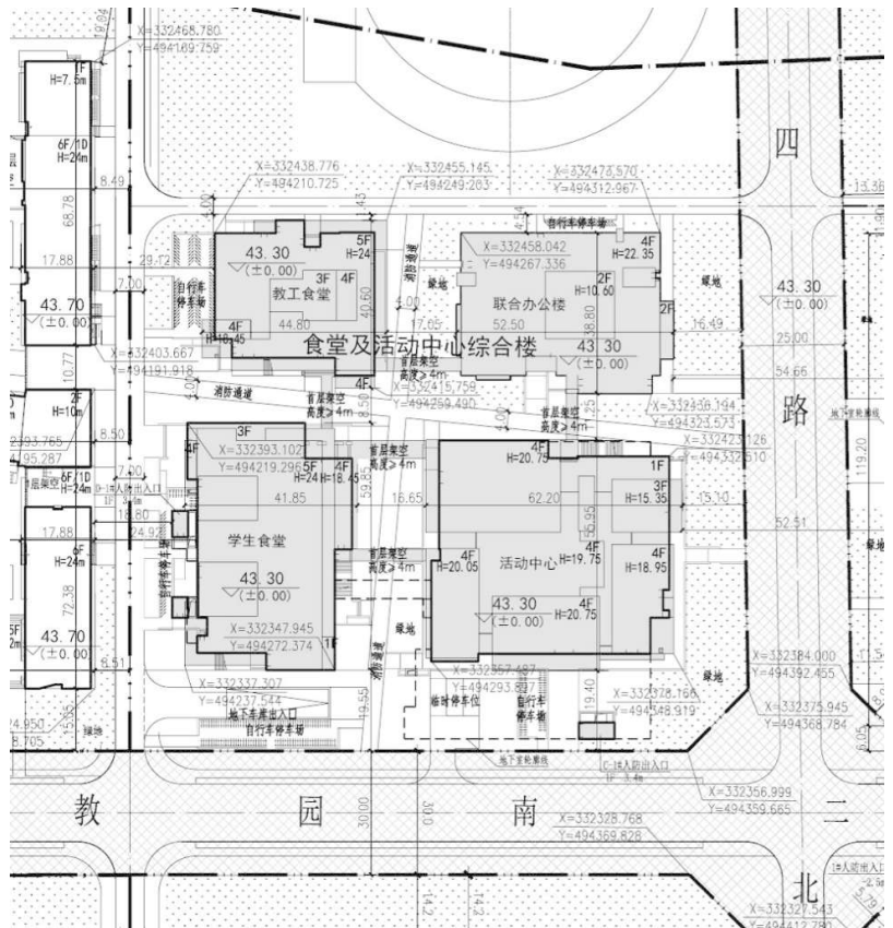
总平面图
