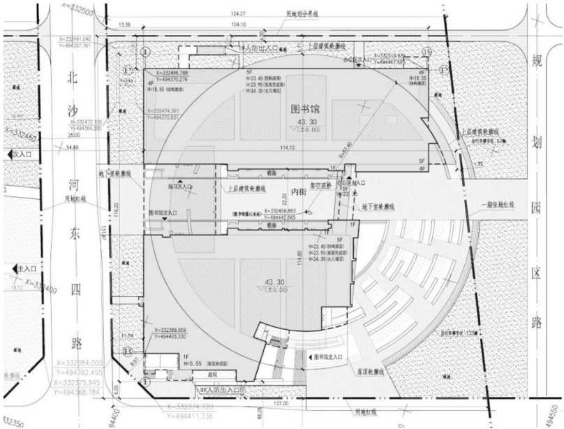
总平面图
