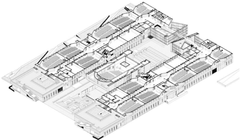
剖轴测图
