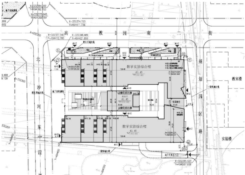
总平面图
