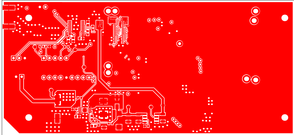
Top Layer (Scale 1:1)
