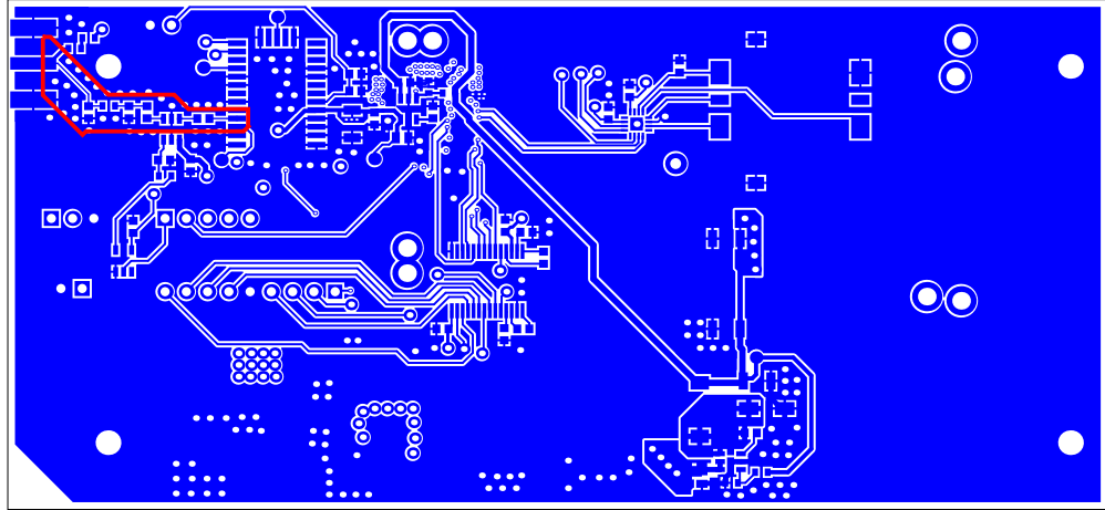
Bottom Layer (Scale 1:1)
