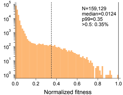
TrpB
