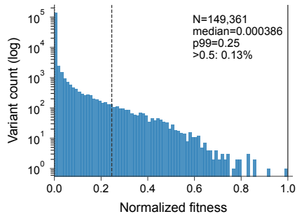
GB1
