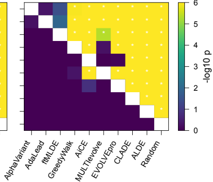
PAB1
