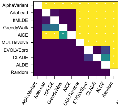
AAV
