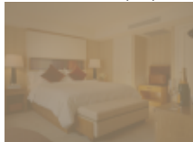
contrast (s3)
