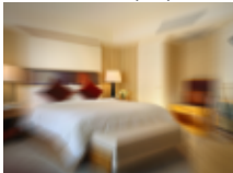
zoom (s3)
