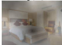
fog (s3)
