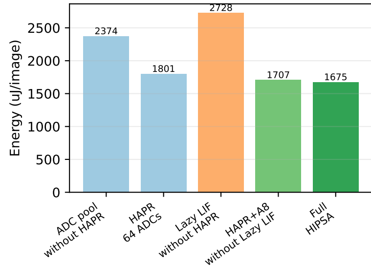
CIFAR10DVS
