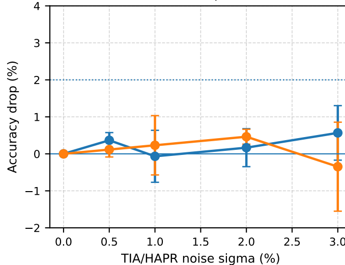
TIA/HAPR output noise
