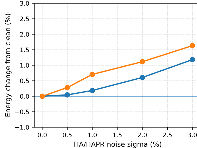
TIA/HAPR output noise
