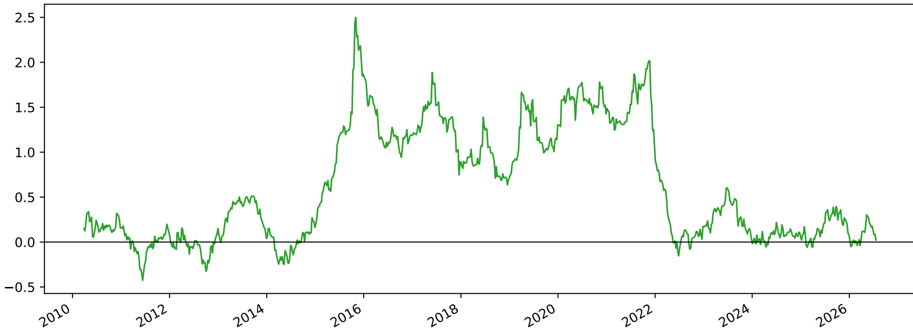
Rolling ICIR (26-week) — IS-model scores
