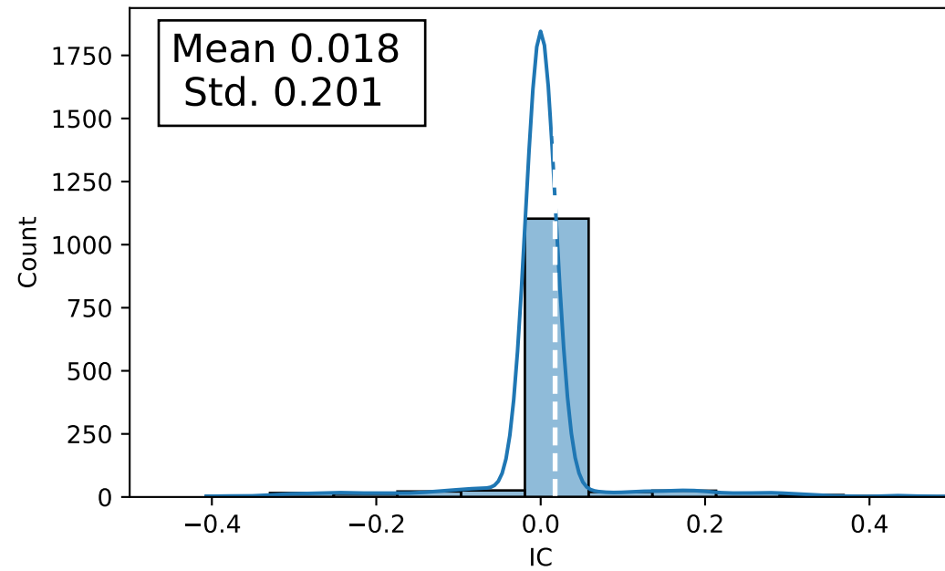
5D Period IC
