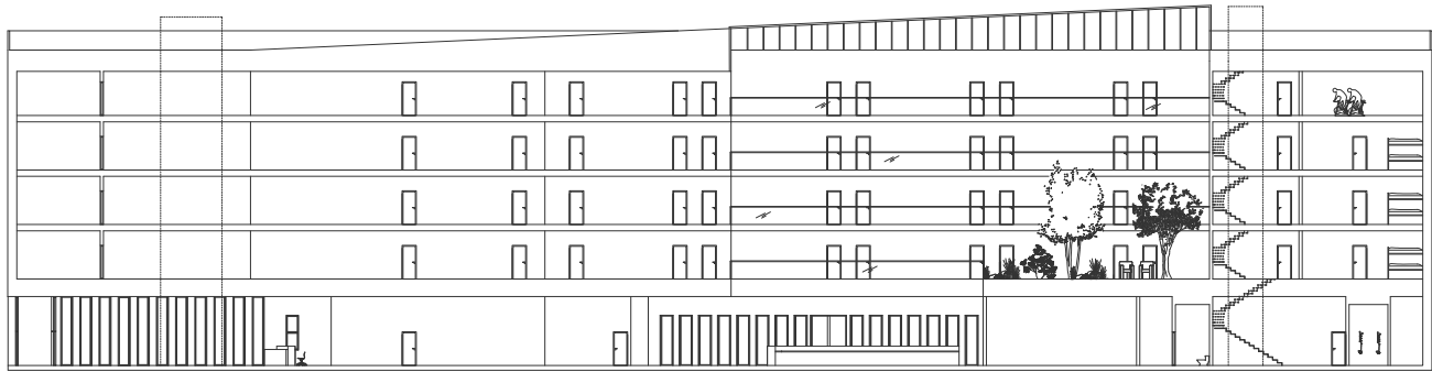
SEKTION B-B 1:200 (A1) Centralt i byggnaden finns ett stort atrium som ger ljus till rumsvåningarnas korridorer och restaurangens bar. På första våningen finns en vinterträdgård som har en visuell förbindelse med restaurangen på bottenplan.
