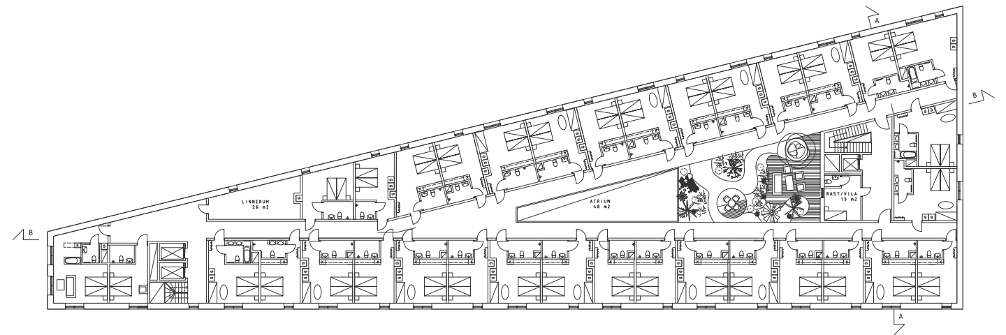
PLAN 1-4 1:200 (A1) Suiter placerats i byggnadens spets med utsikt mot Älvsborgsbron, rymliga handikappersrum i hörnen och en ett vilrum för städpersonal i den bredaste delen intill atriumet.
