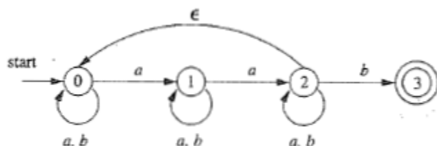
图 3-29 练习 3.6.3 的 NFA
