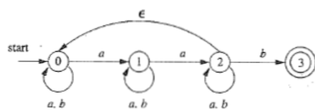
图 3-29 练习 3.6.3 的 NFA
