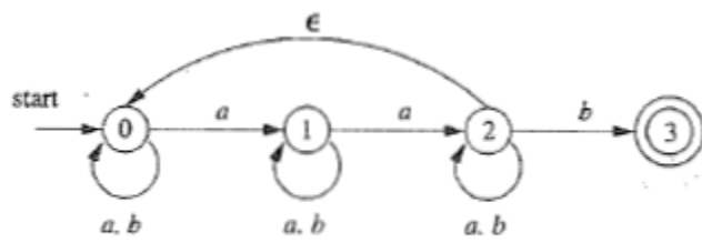
图 3-29 练习 3.6.3 的 NFA
