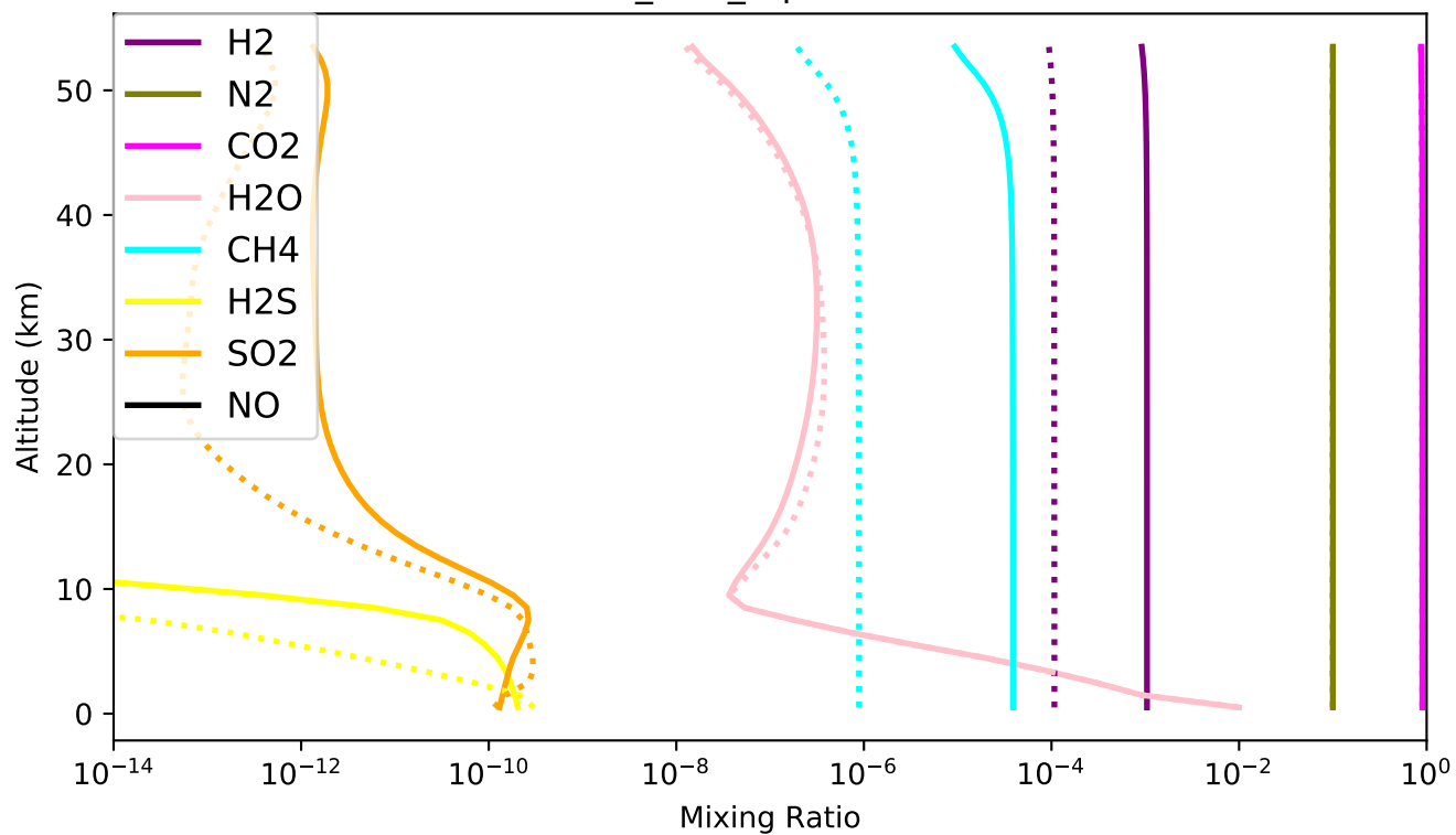
Sun_CO2_reproduction
