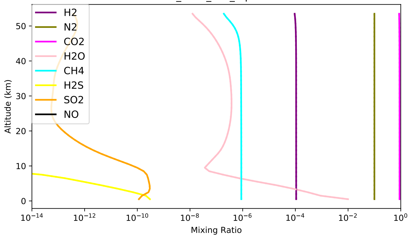
scenario_CO2r_emi_reproduction
