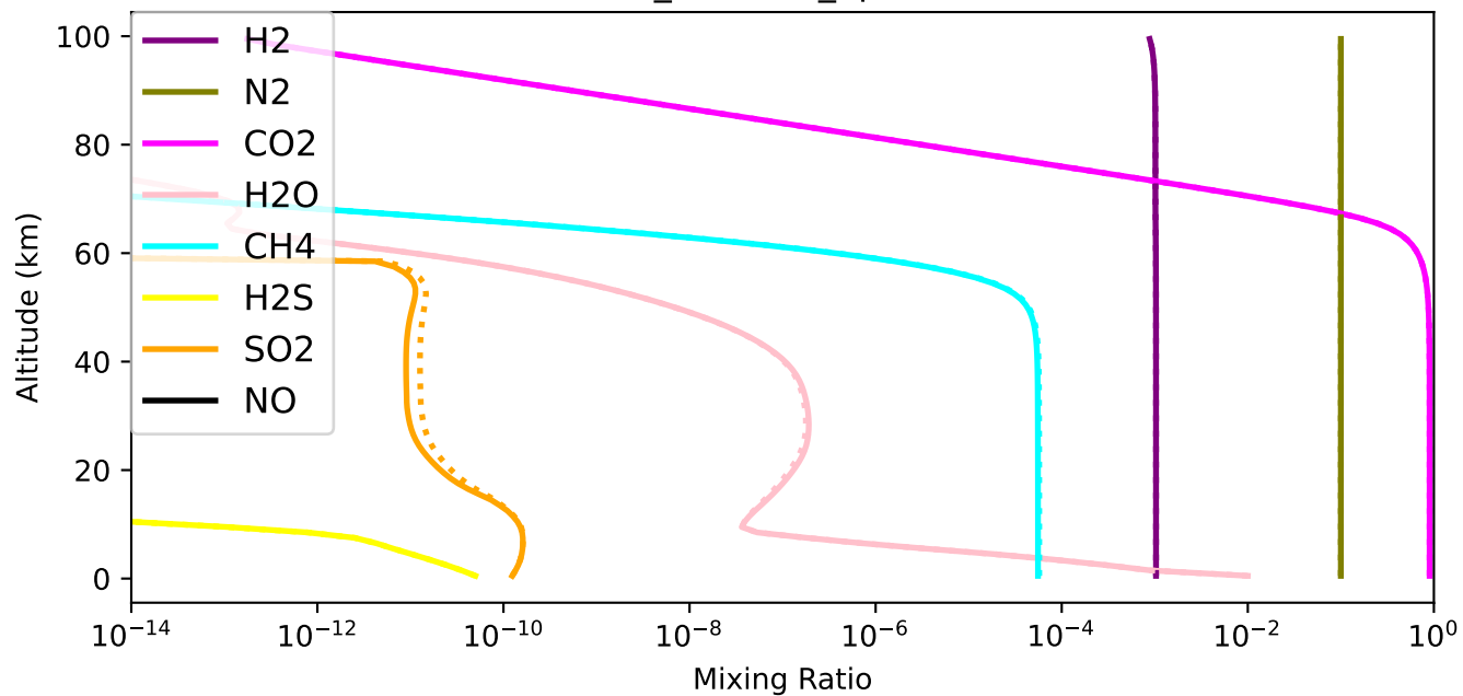
Sun_CO2-Full_updates
