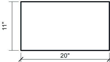
2 SIDE PANEL 0.75" THK · ×2
