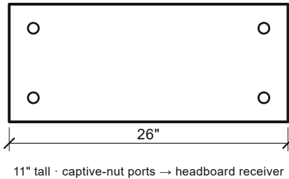
3 BACK PANEL 0.75" THK · ×1
