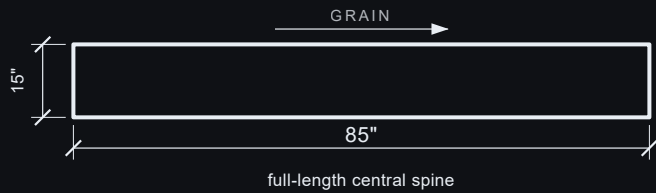
2 CENTER SPINE 3" THK · ×1
