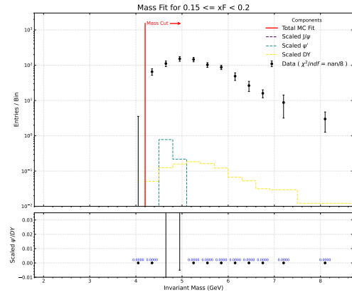
(d) 0.15 \leq x_F < 0.2
