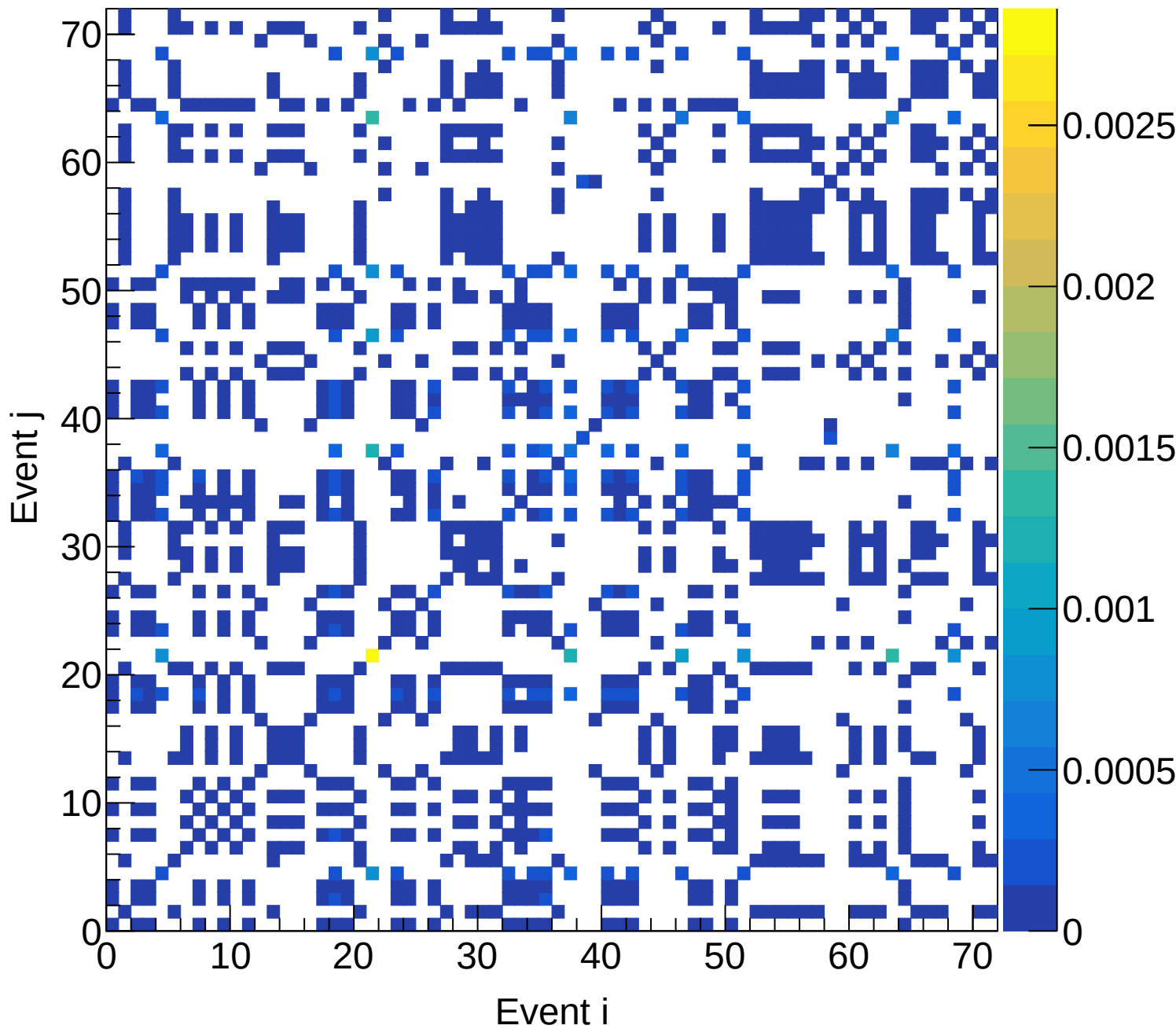
LH2 (total) Covariance | M: [5.1, 5.4) xF: [0.00, 0.05)
