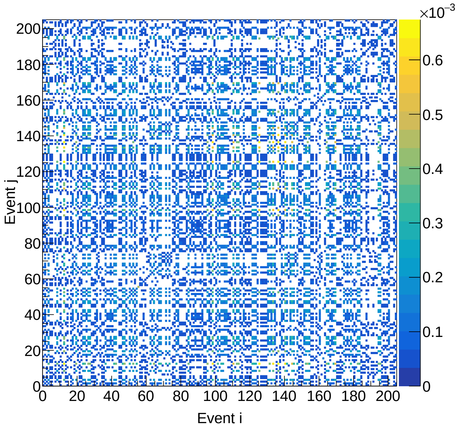
LH2 (total) Covariance | M: [5.1, 5.4) xF: [0.15, 0.20)
