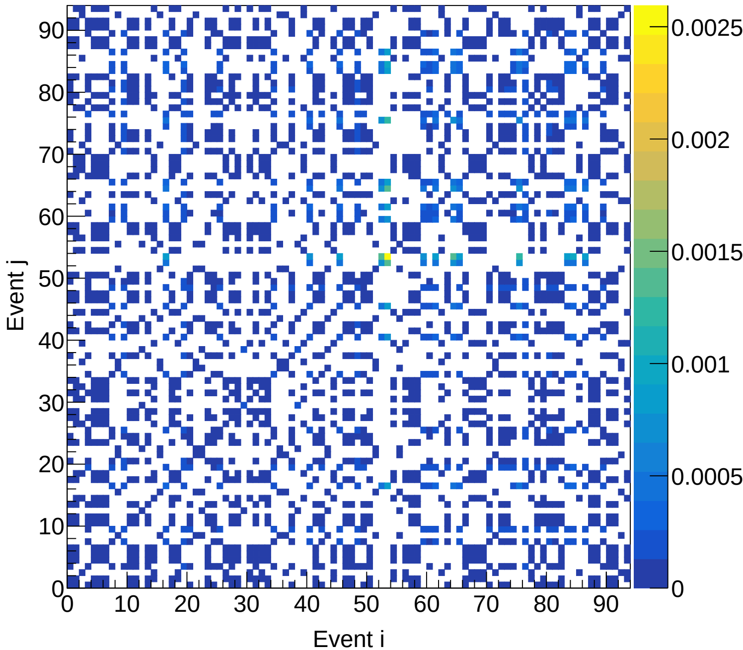
LH2 (total) Covariance | M: [5.7, 6.0) xF: [0.15, 0.20)
