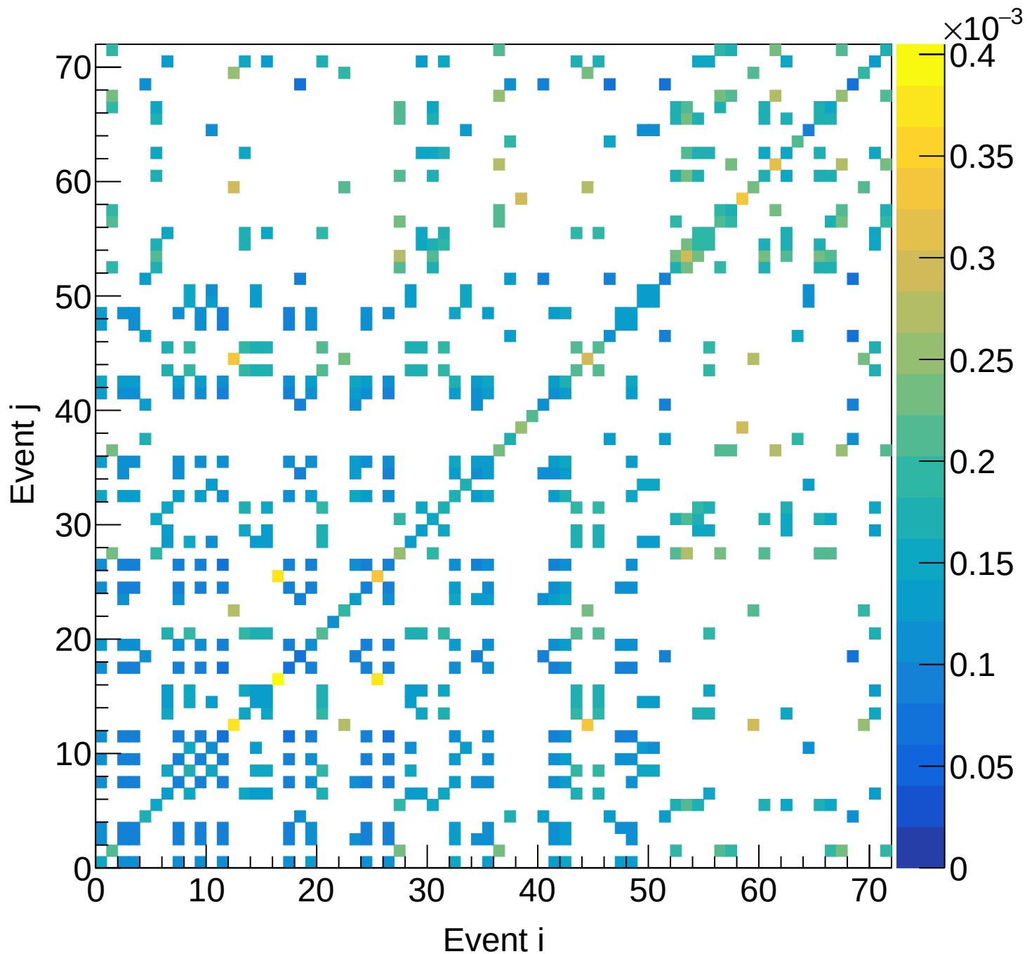
LH2 (total) Covariance | M: [5.1, 5.4) xF: [0.00, 0.05)
