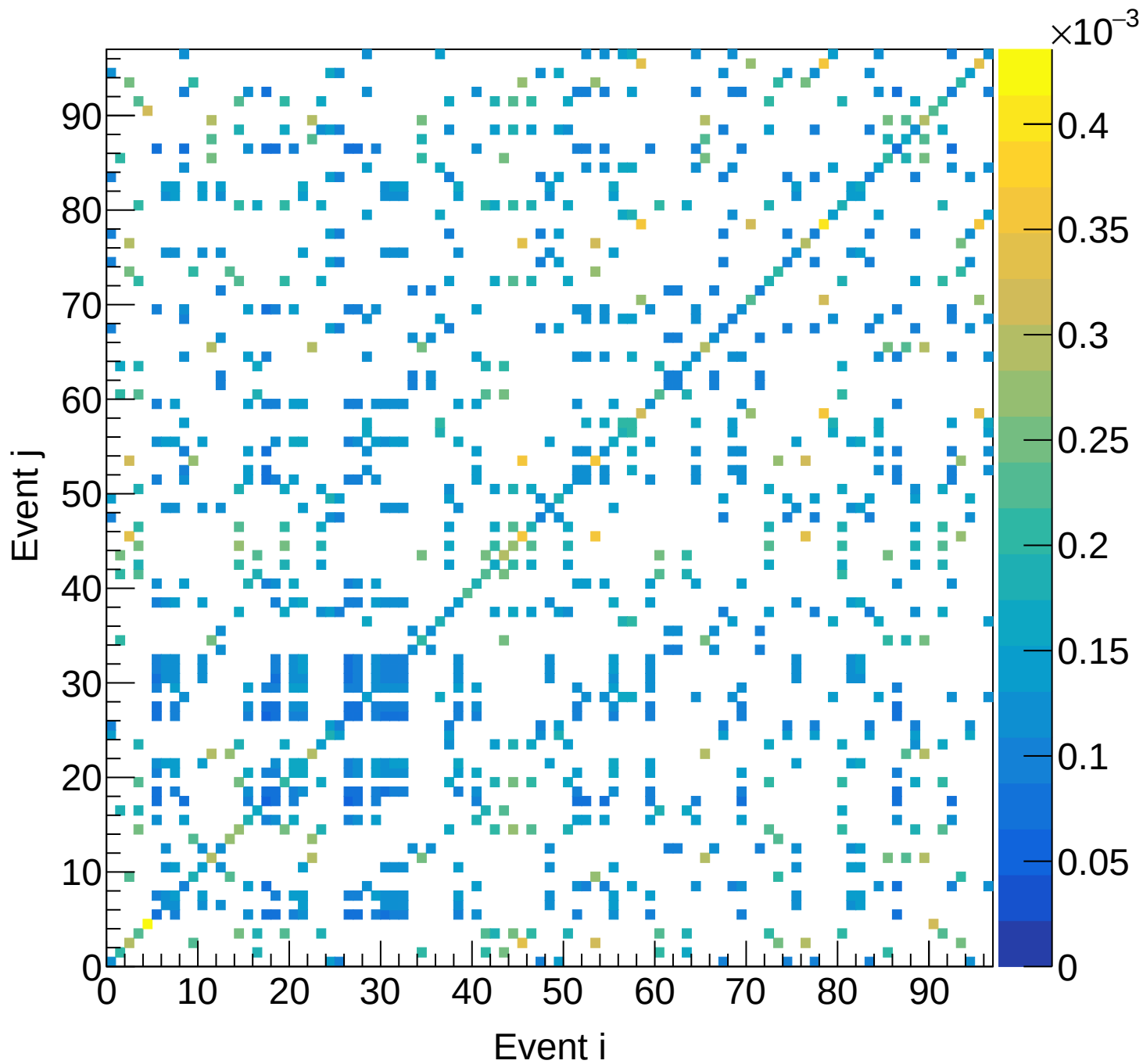
LH2 (total) Covariance | M: [5.1, 5.4) xF: [0.05, 0.10)
