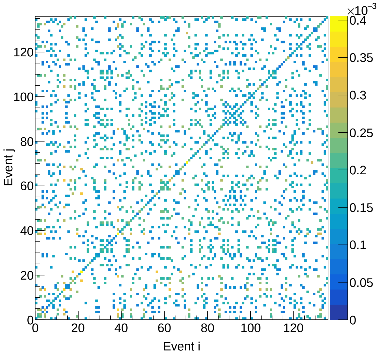
LH2 (total) Covariance | M: [5.1, 5.4) xF: [0.10, 0.15)
