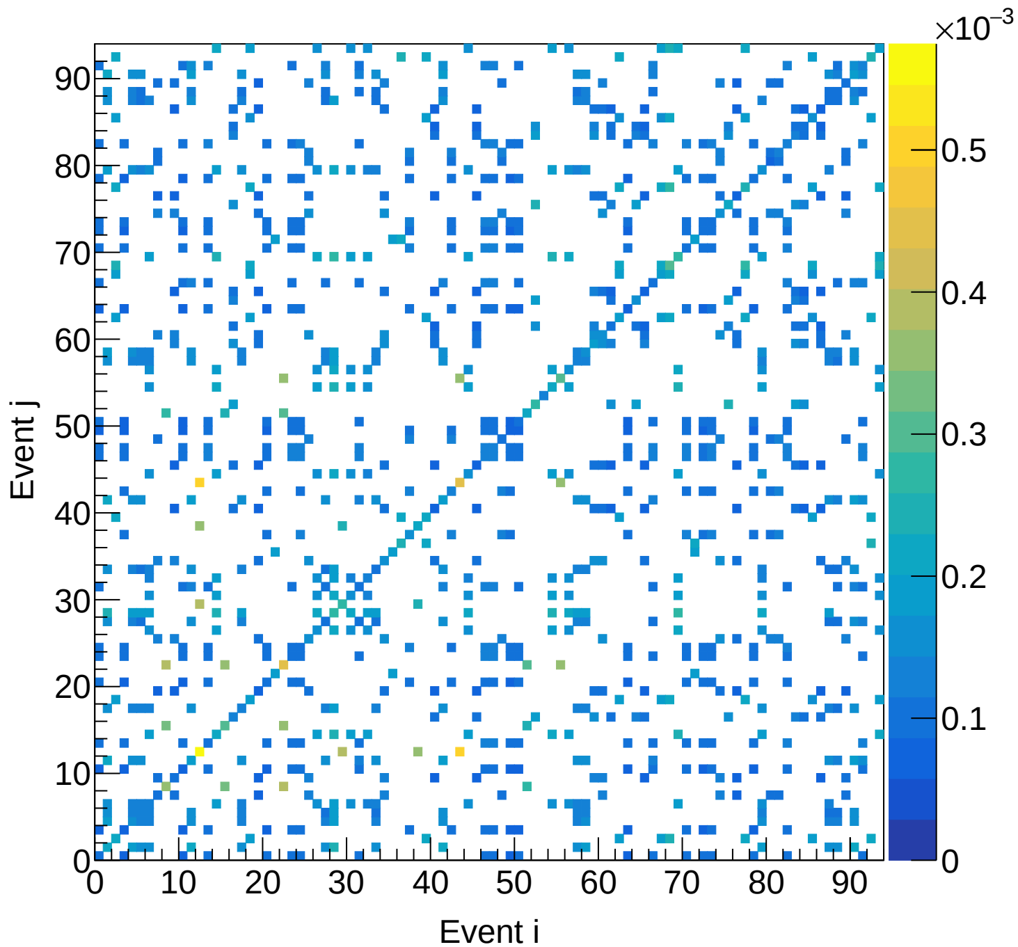
LH2 (total) Covariance | M: [5.7, 6.0) xF: [0.15, 0.20)
