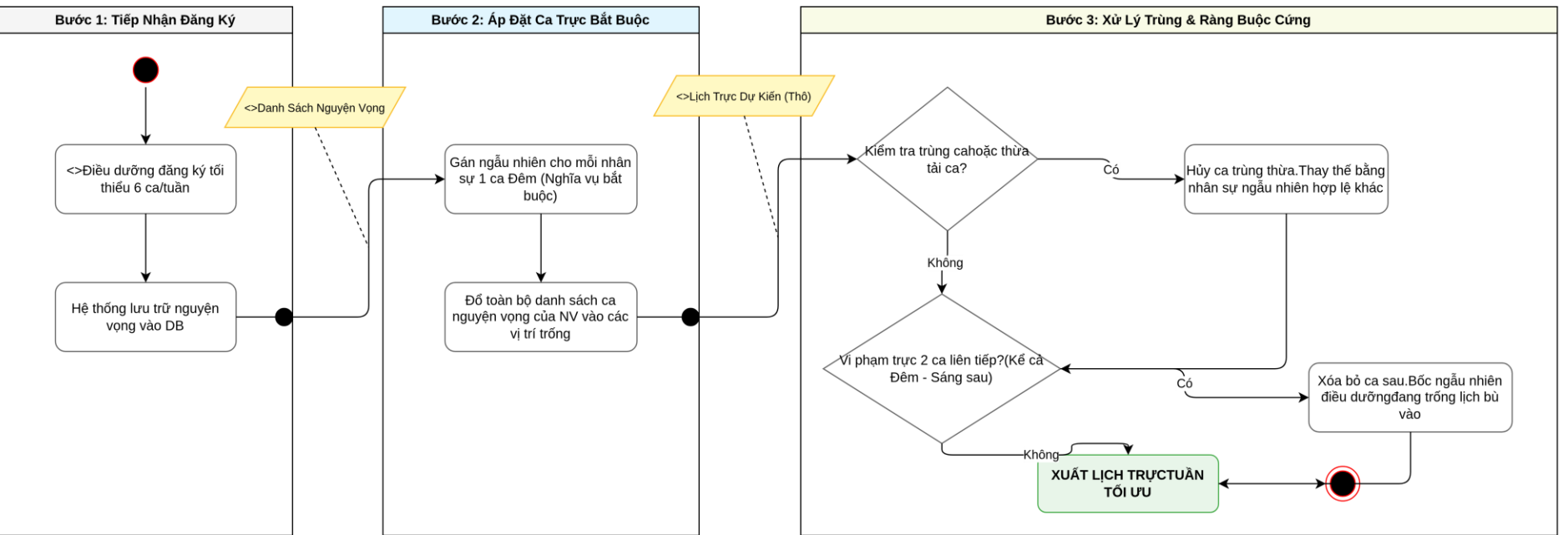
HỆ THỐNG TỰ ĐỘNG XẾP LỊCH TRỰC ĐIỀU DƯỠNG (ALGORITHM FLOW)
