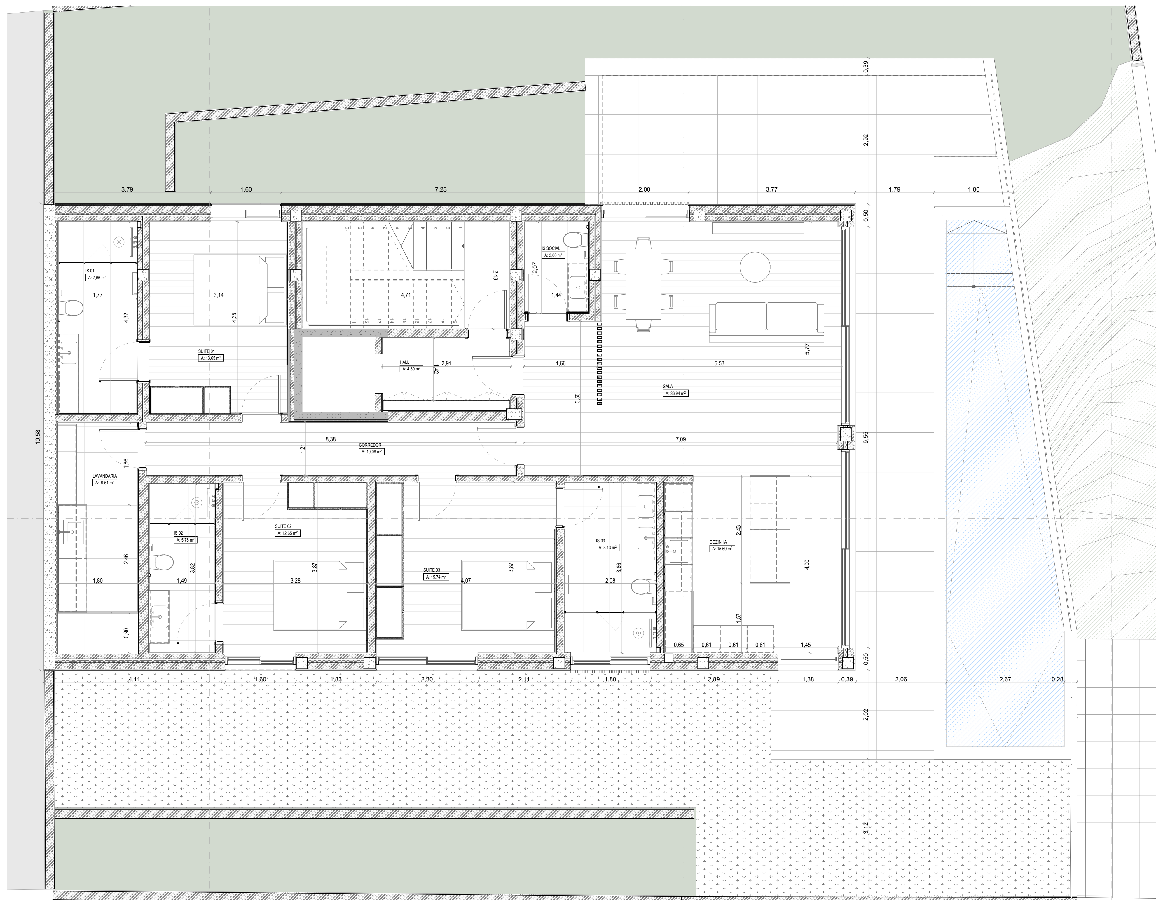
PLANTA PISO 1 1:50 FRAÇÃO A
