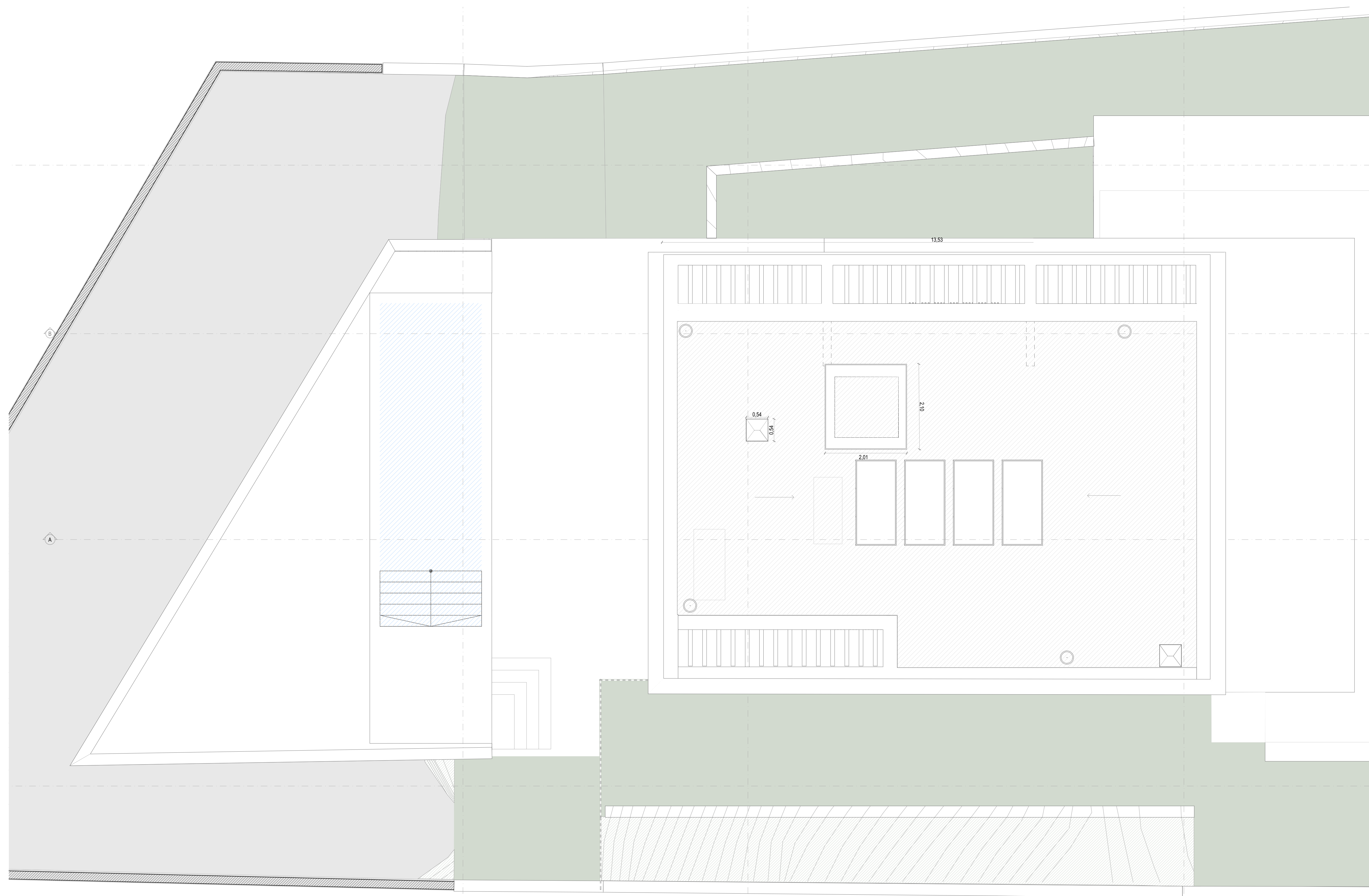
PLANTA DA COBERTURA 1:50
