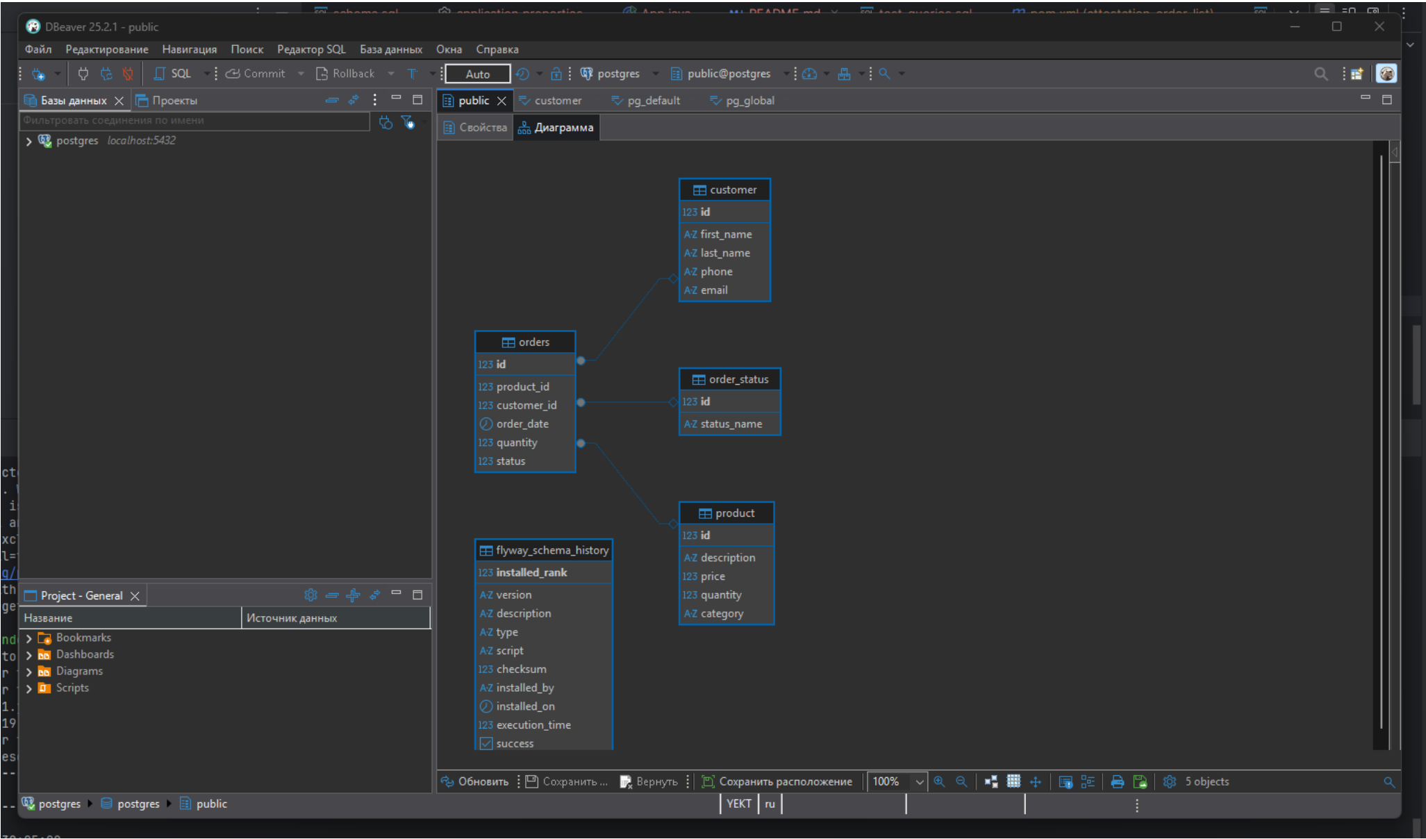
Диаграмма - DBeaverDiag.png / смотреть
