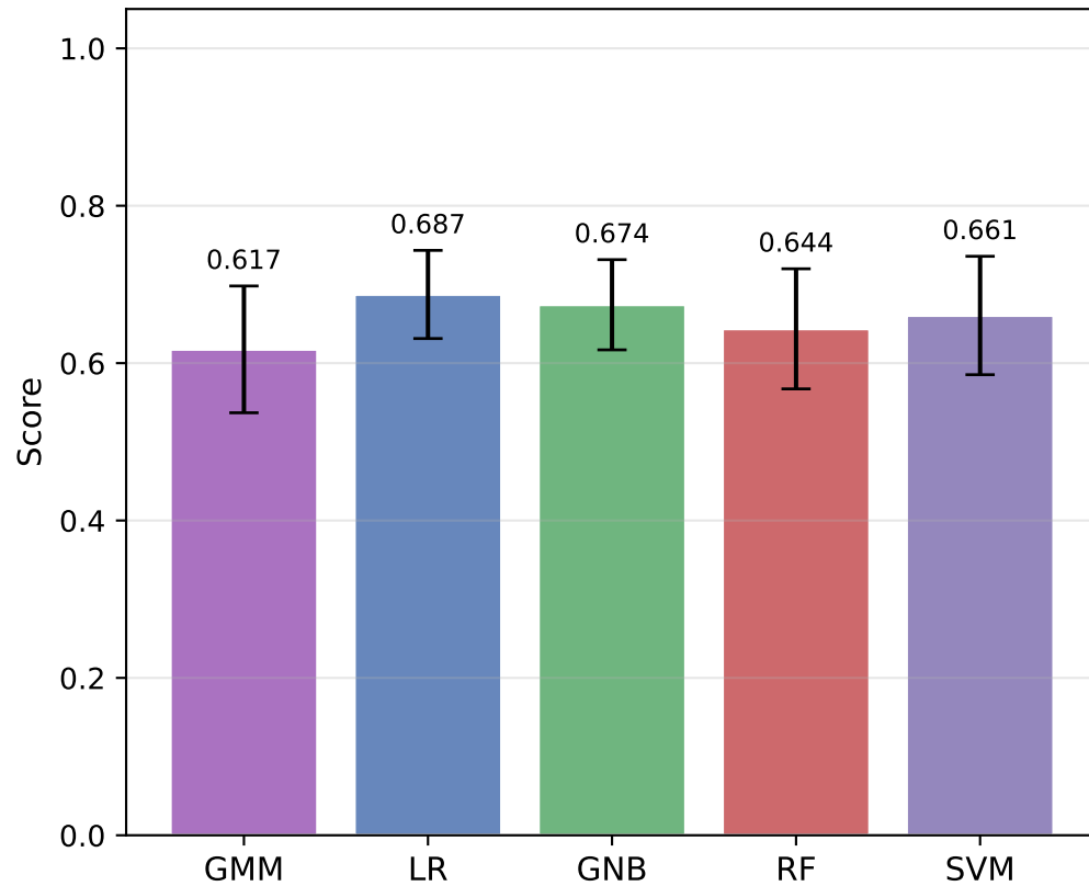
F1 Score
