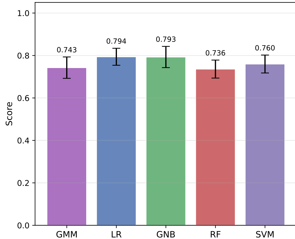
AUC-ROC
