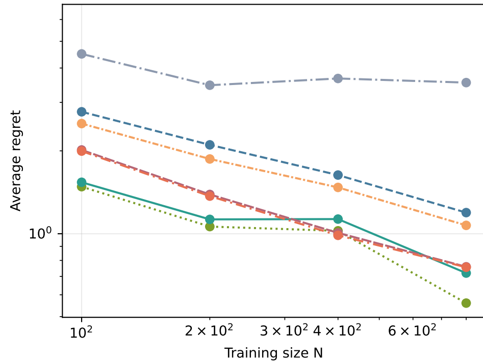
Benchmark A: d=5, k=3
