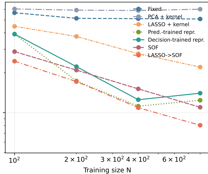
Benchmark A: d=100, k=3
