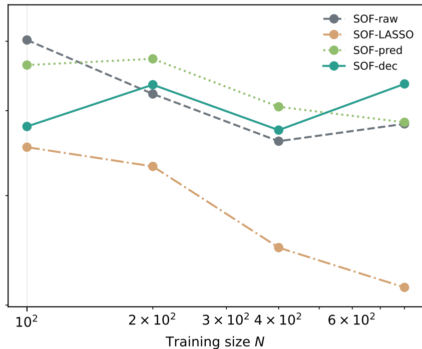
Benchmark A: (d, k) = (100, 3)
