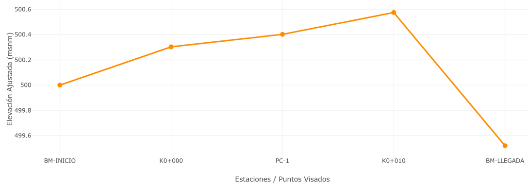
Figura 1: Perfil altimétrico de la línea de nivelación compensada
