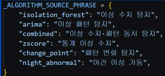
< 알람 팝업창 원인별 메세지 매핑 >
