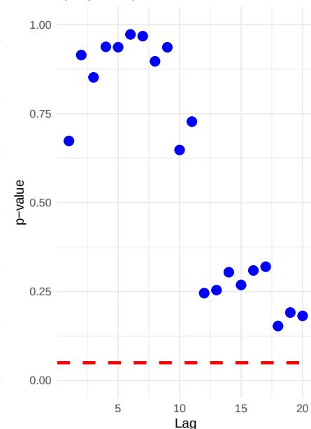
Ljung-Box p-values
