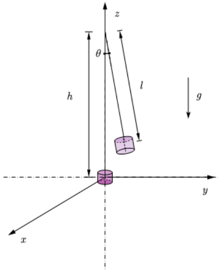
图8 单磁铁体系仪器图
