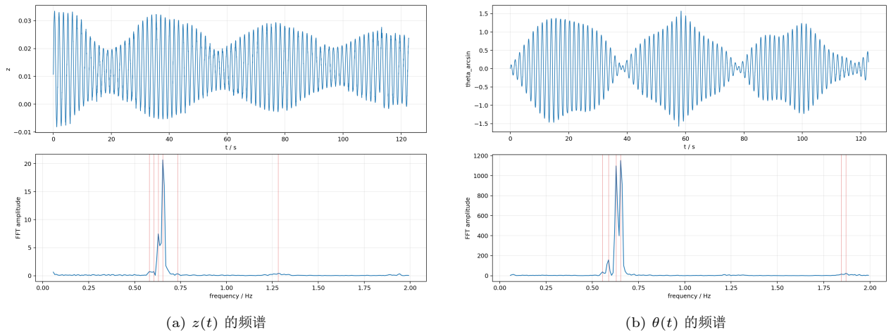
图 5: 强耦合数据的傅里叶分析。
