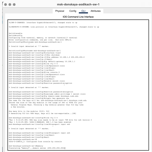
Рис. 2: Настройка коммутатора
