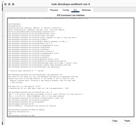
Рис. 5: Настройка коммутатора
